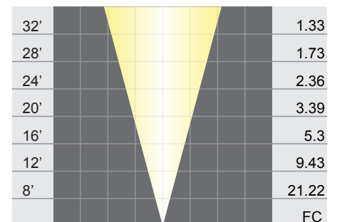
PAR36 LED: LED-7W-CPFL27K
